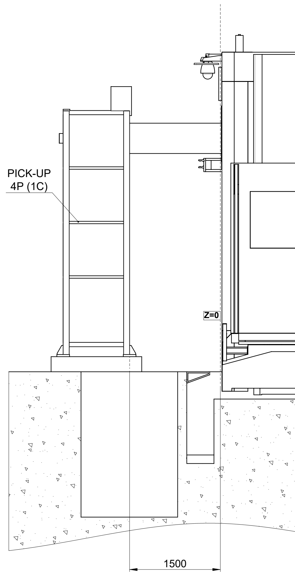
A-A 270°
